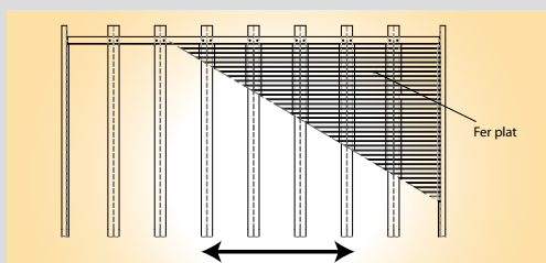
Structure renforcée
